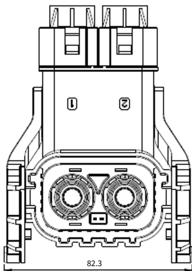
弯头插头外形图
