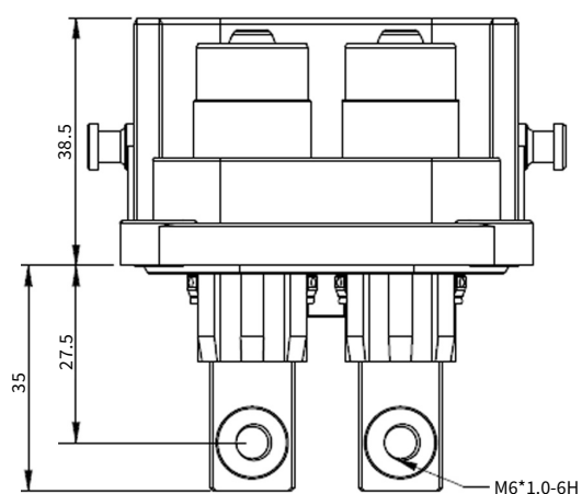
180度铜排引出方式
