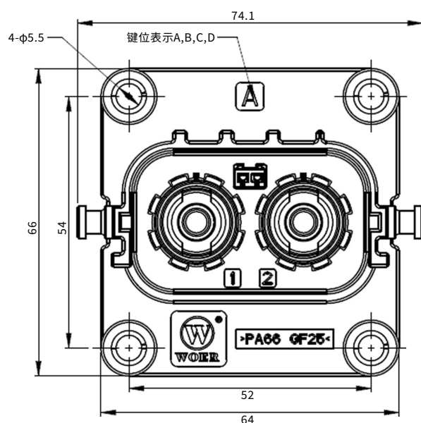
插座外形图
