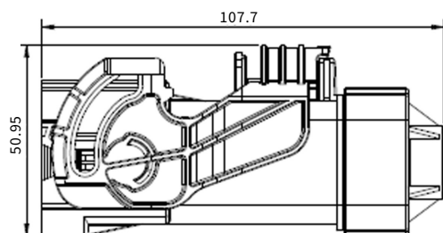
直头插头外形图
