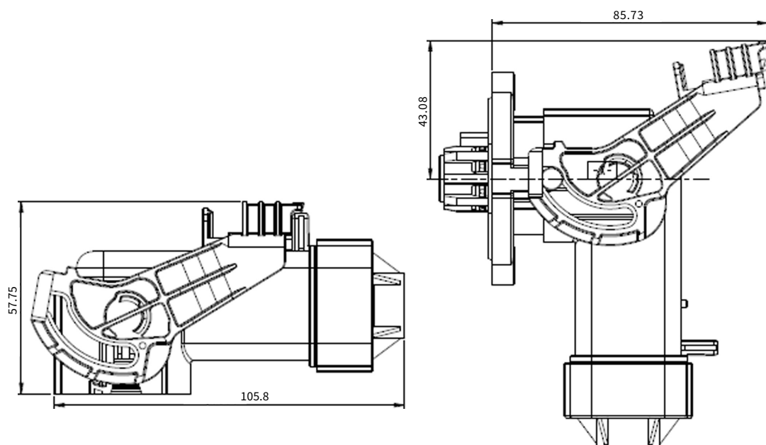
插头与插座互配, 手柄开启状态
